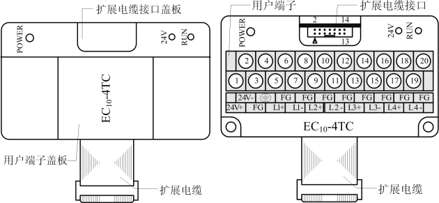
图 1-1 模块接口外观图
