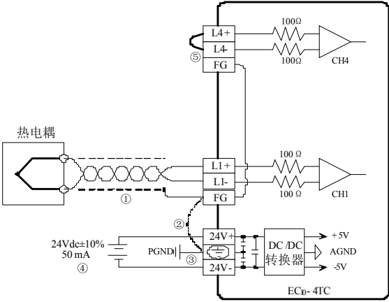
图 1-4 用户端子布线示意图
