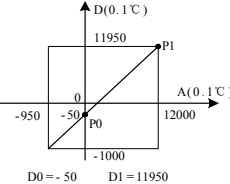
图 3-3 特性更改举例
